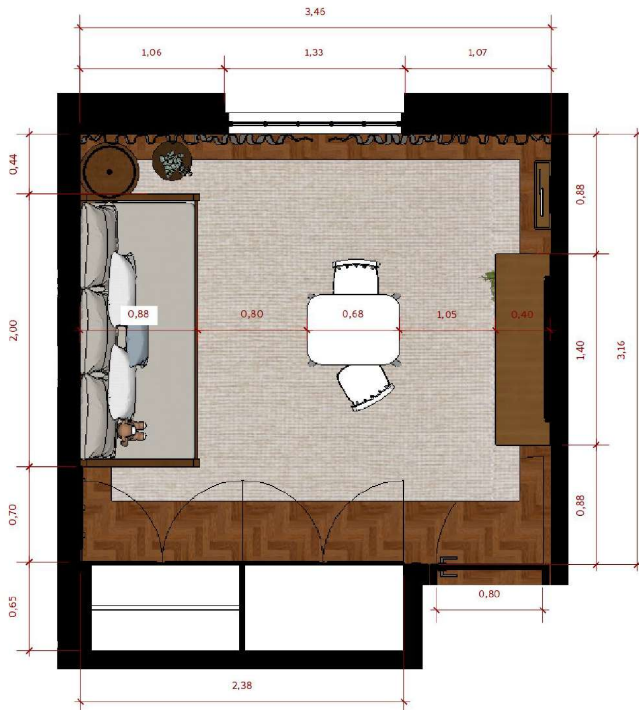
DORMITÓRIO ALICE. planta baixa R02
